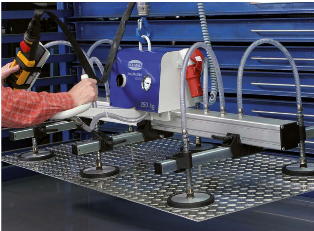
Bild 5-4: Traverse mit Saugtellern nimmt nicht magnetisierbare Blechtafel auf
