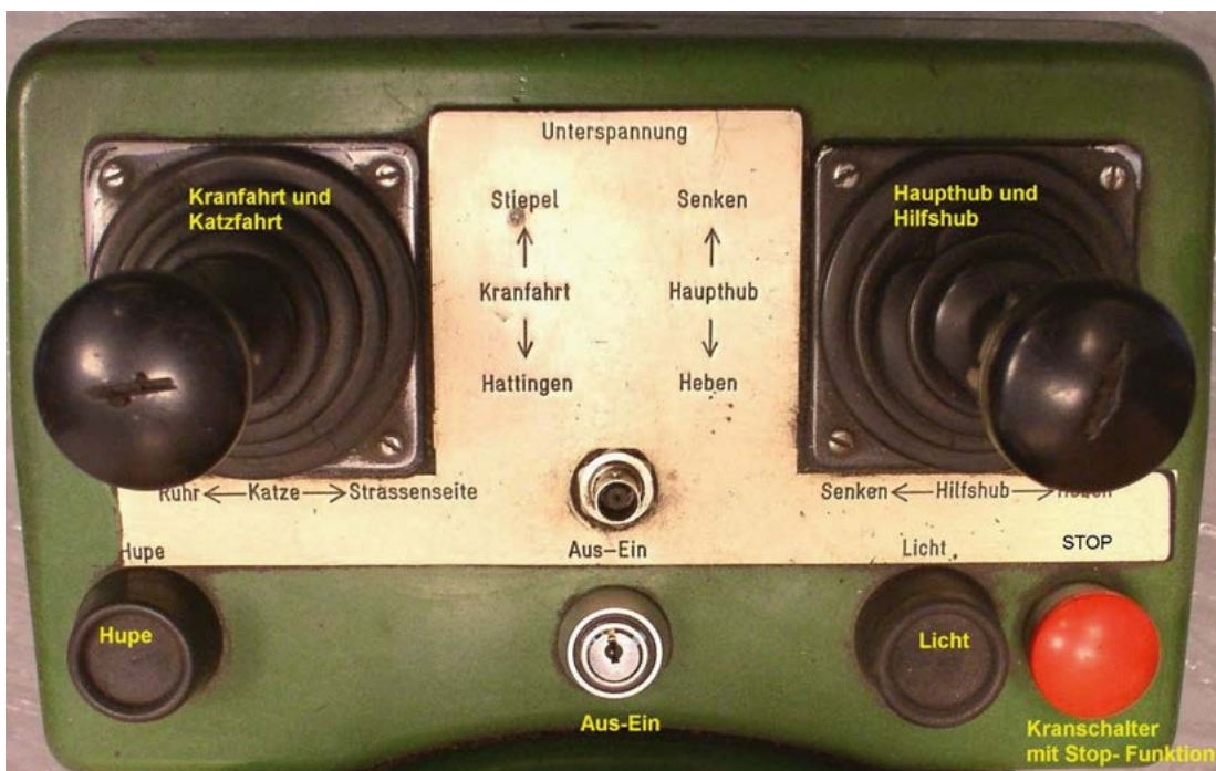
Bild 3-4: Steuergerät einer Funksteuerung mit Zuordnung der Stellteile. Zur Sicherung gegen unbeabsichtigtes Betätigen sind die Stellteile mit „Totmannschalter“ ausgerüstet; möglich sind z. B. auch Schutzbügel oder vertieft angeordnete Stellteile (siehe auch Bild 4-10)
